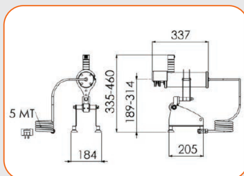
Dimension TS-01
